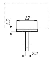
poręcz płaska flat handrail
