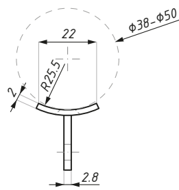
poręcz okrągła round handrail
